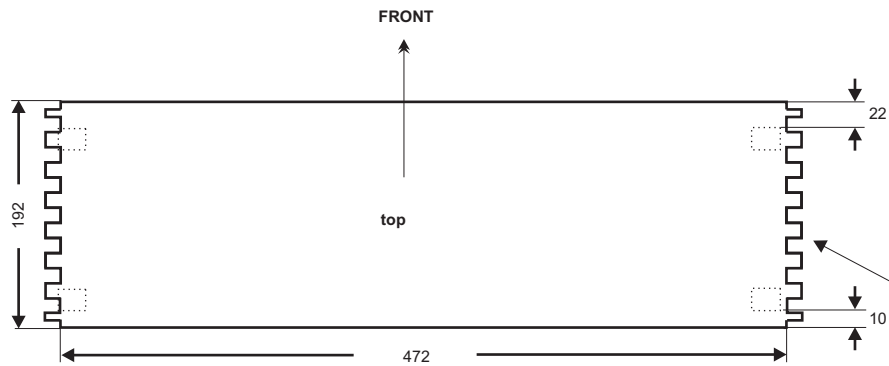
10er finger joints
